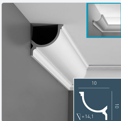
Orac Luxxus C902
