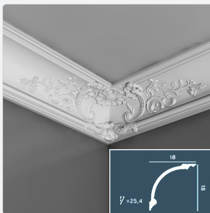
Orac Luxxus C338B (угол)
