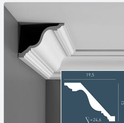
Orac Luxxus C334
